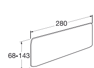
Торцева заглушка для системних підвіконь з нарощеним капіносом
