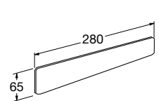
Торцева заглушка для системних підвіконь з нарощеним капіносом
