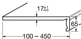
Системне підвіконня compact-blende з подовженим капіносом
